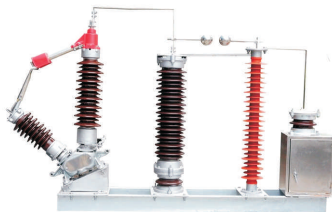
GW13-110
