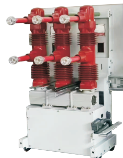
SF6-40.5
