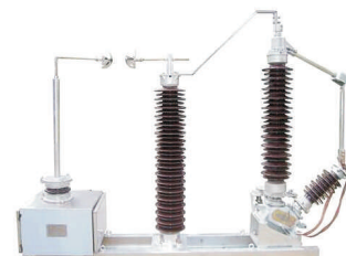
GW13-220
