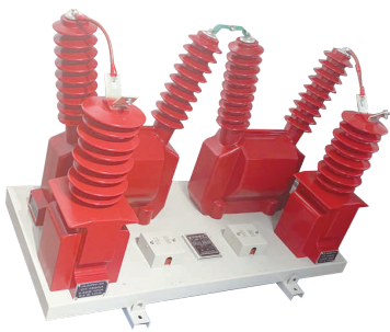
JLSZV-35W
