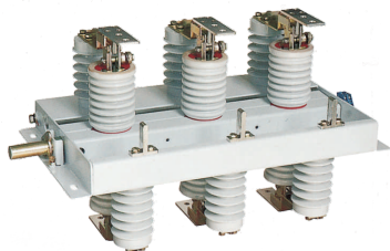
GN30-12(D)
