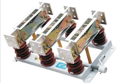
GN22-12(CD)
